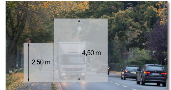
Lichtraumprofil
